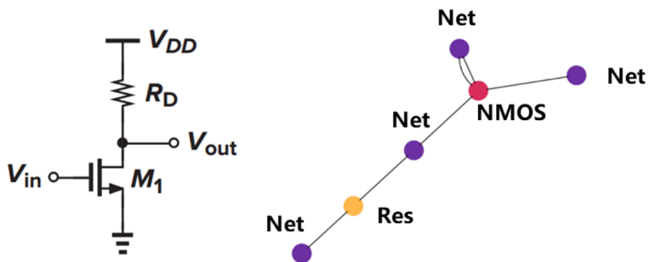
图 4: 图片转 graph 示意
