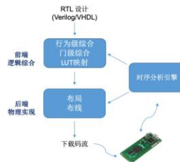
图四 FPGA EDA 流程
