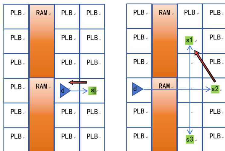
图五 通过单元移动的详细布线优化
